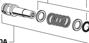
912647-0070A CAP SEAL
